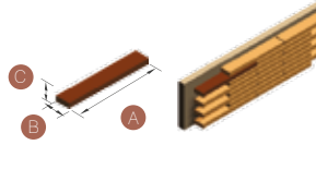
Selçuklu (Çubuk) Pres Tuğla / Seljuk (SPT/3) Ebatlar / dimensions : 300 x 35 x 20
