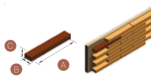
Selçuklu (Çubuk) Pres Tuğla / Seljuk (SPT/2) Ebatlar / dimensions : 300 x 50 x 30
